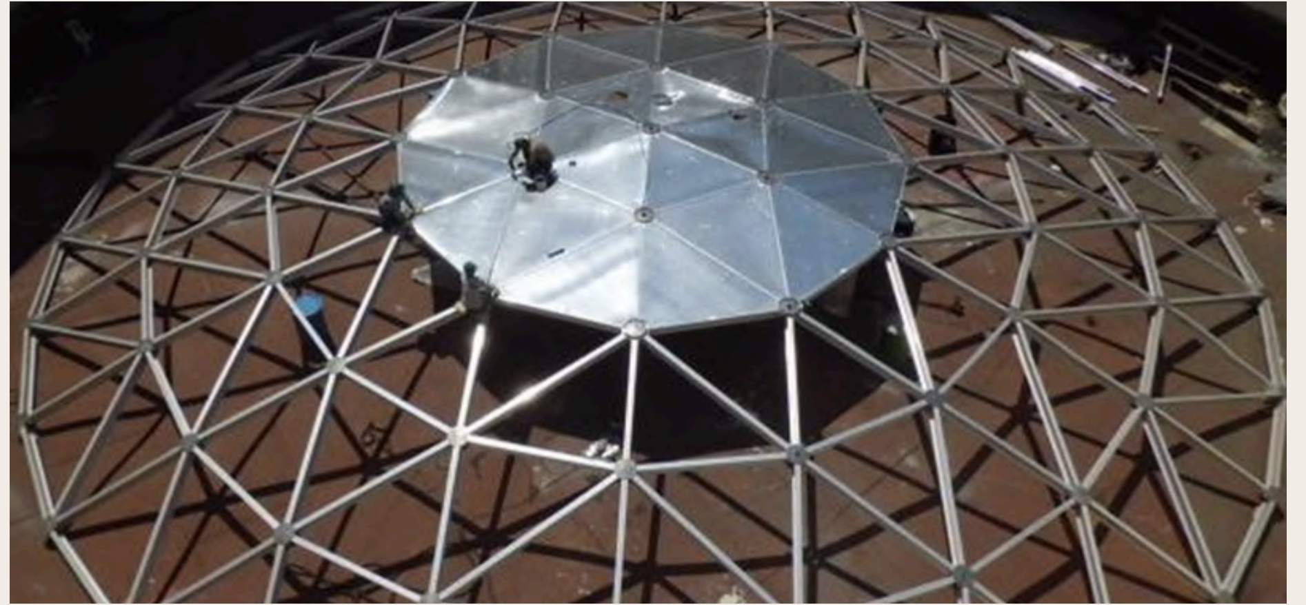
ALUMİNYUM KUBBE ÇATI İMALATI
